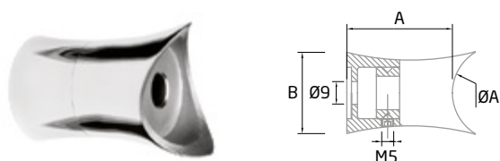
ST-313 AISI-316
