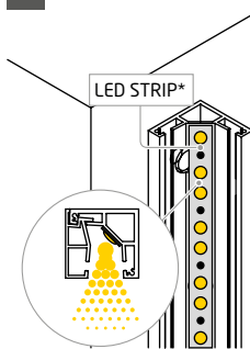
3 Colocación tira LED
