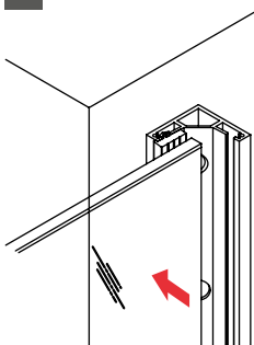
5 Instalación del vidrio
