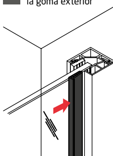
7 Fijación del vidrio con la goma exterior
