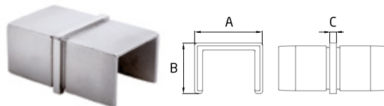
CT-241 AISI-316
