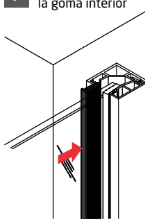
7 Fijación del vidrio con la goma interior
