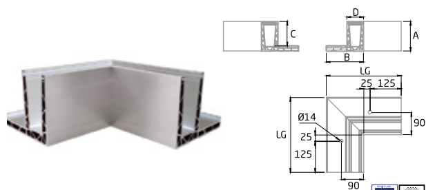
SV-1703-C INSIDE
