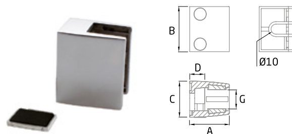
CC-738 AISI-316
