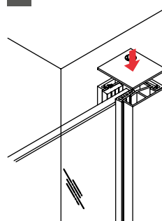
8 Colocación de la tapa superior
