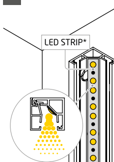
3 Colocación tira LED
