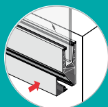
Perfil en "U" con aleta (perfil en "Y")
