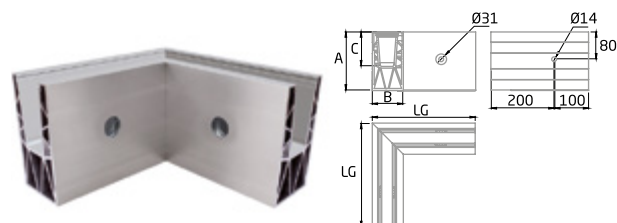
SV-1802-C INSIDE
