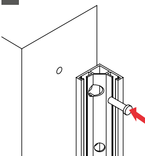
2 Anclaje parte 1
