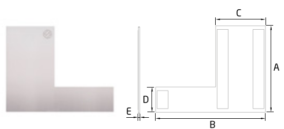
EC-1703-3
