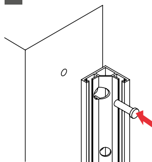
2 Anclaje parte 1
