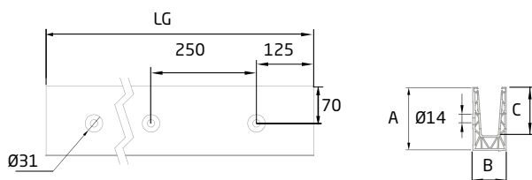
SV-1702
