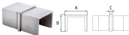
CT-241 AISI-316
