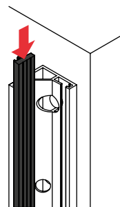
4 Mise en place du joint intérieur.
