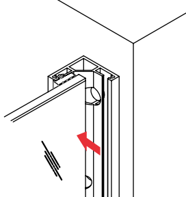
5 Installation du verre.
