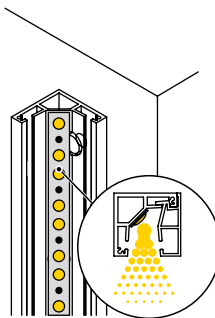
3 Mise en place du ruban LED.
