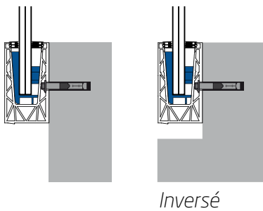
Profilé en « U » latéral
