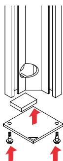
1 Fixation du cache inférieur.
