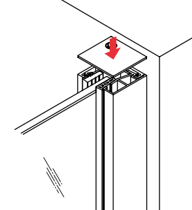
8 Mise en place du cache supérieur.
