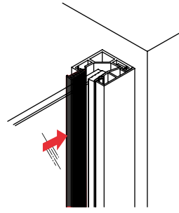
7 Fixation du verre avec le joint extérieur.
