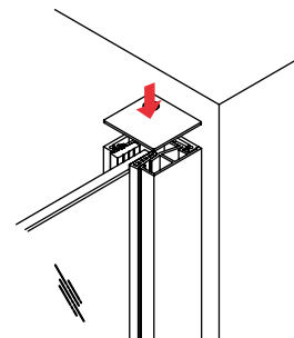
8 Mise en place du cache supérieur.
