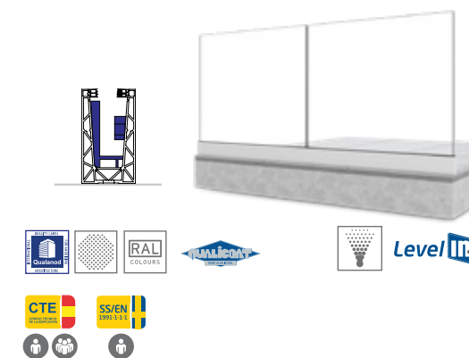
Système GlassFit Flow SV-1701 Top
