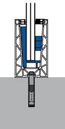
Profilé en « U » supérieur
