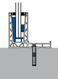
Profilé en « F » supérieur
