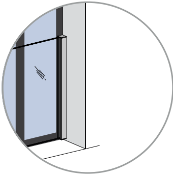
Sur le cadre de la menuiserie
