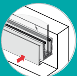
Profilé en « U » inversé (côté inversé)
