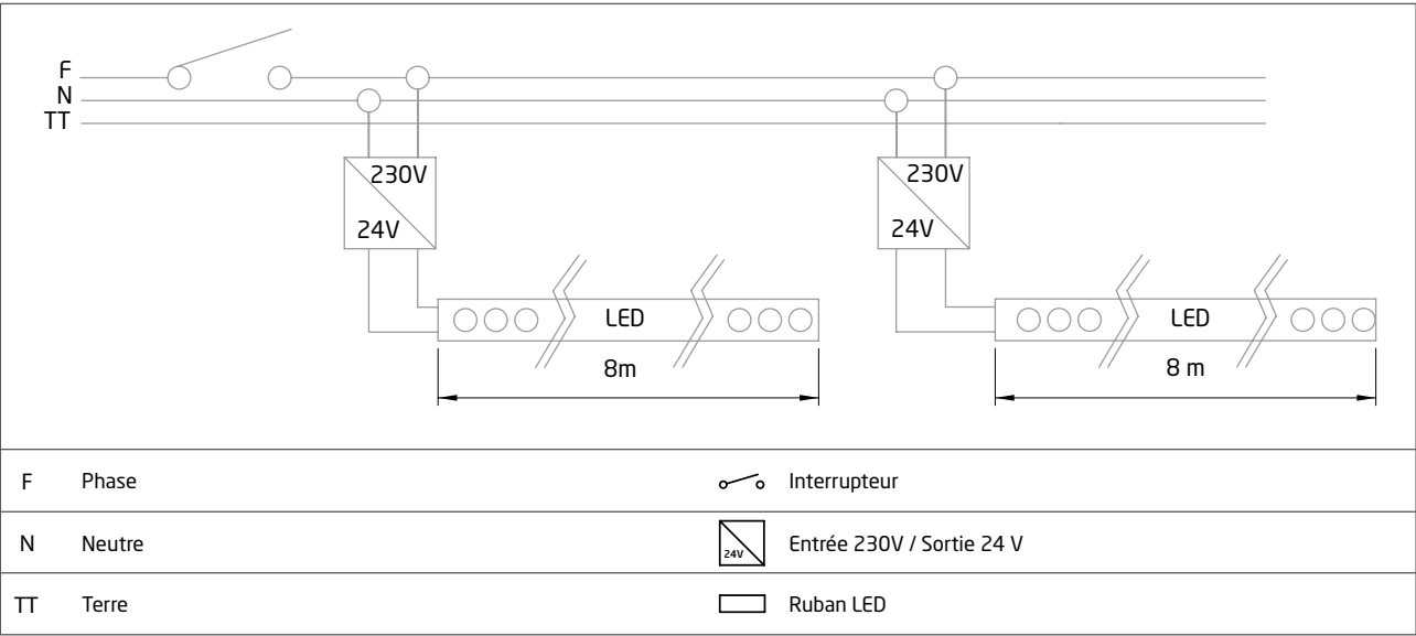
Schéma de raccordement
