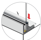
Profilé en « U » avec aile (profilé en « F »)
